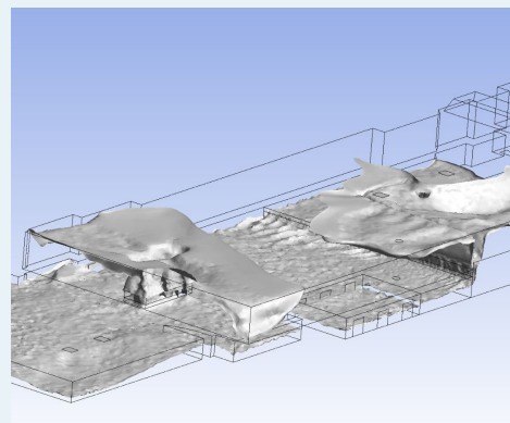
Accompagnement en simulation de désenfumage
